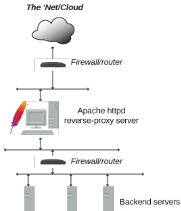
Figura 3. Proxy reverso no Apache [Apache 2020].
