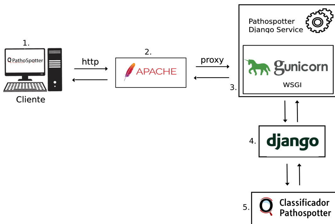
Figura 4. Arquitetura do PathoSpotter Classifier .
